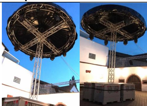
PilzTruss PT-4,5d,4,5h:
